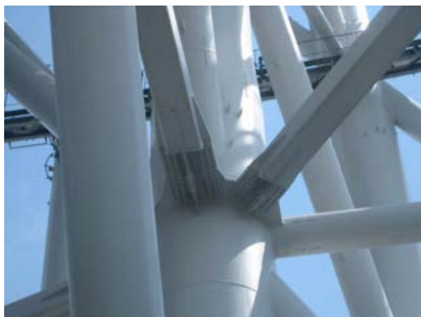
4 階のタワーの構造部
